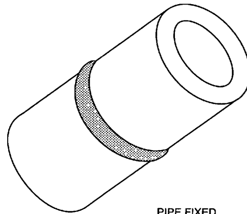
(D) MULTIPLE WELDING TEST POSITION—6GR
