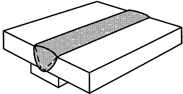
(D) SINGLE-V-GROOVE WELD WITH BACKING
