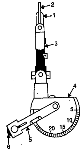
FIG. 14.7. DE LISLE'S CLINOMETER.
