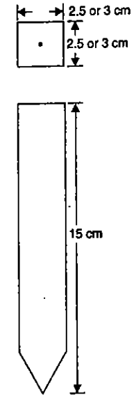
FIG. 3.16. WOODEN PEG.
