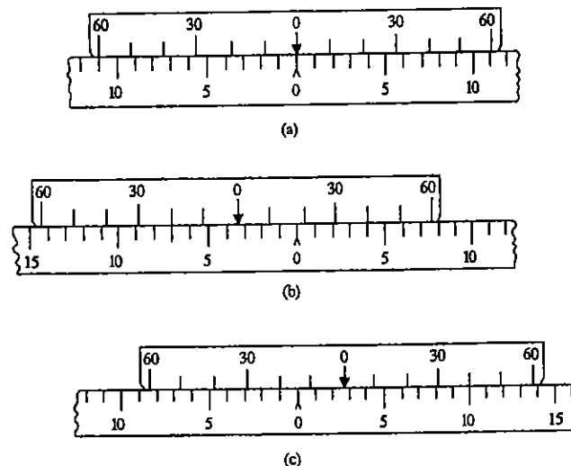
FIG. 1.9 EXTENDED VERNIER.
