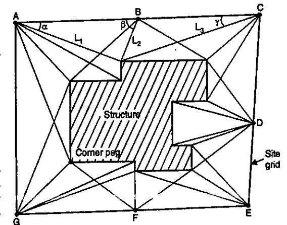
FIG. 20.3. SITE GRID.
