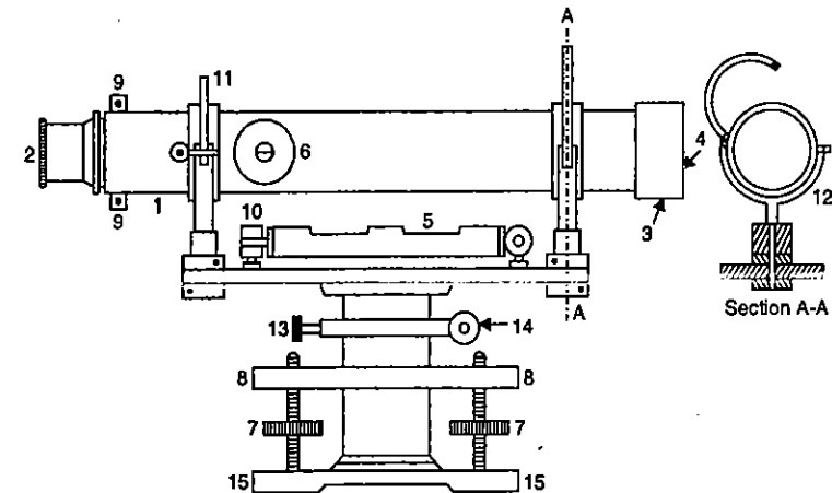
FIG. 9.7. WYE LEVEL.
