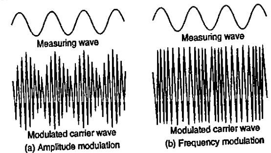
FIG. 24.4. MODULATION
