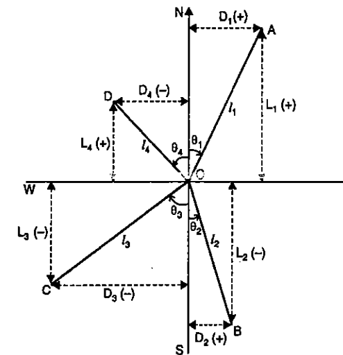
FIG. 8.1. LATITUDE AND DEPARTURE
