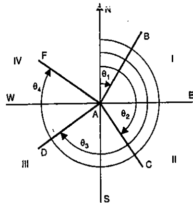
FIG. 5.1 W.C.B. SYSTEM.
