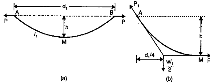
FIG. 3.28. SAG CORRECTION
