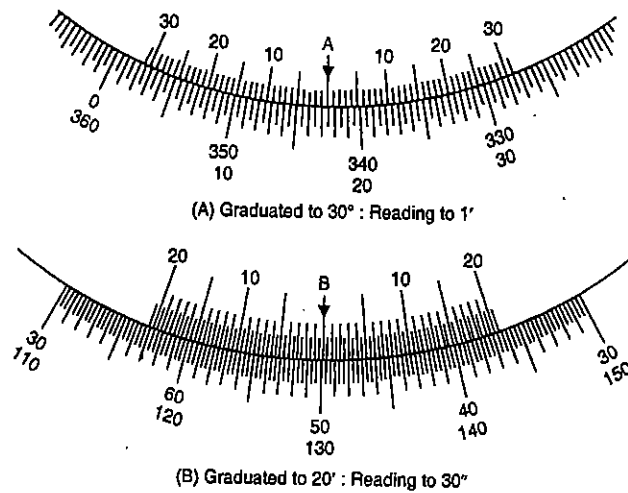
FIG. 1.11. VERNIERS TO CIRCULAR SCALES.
