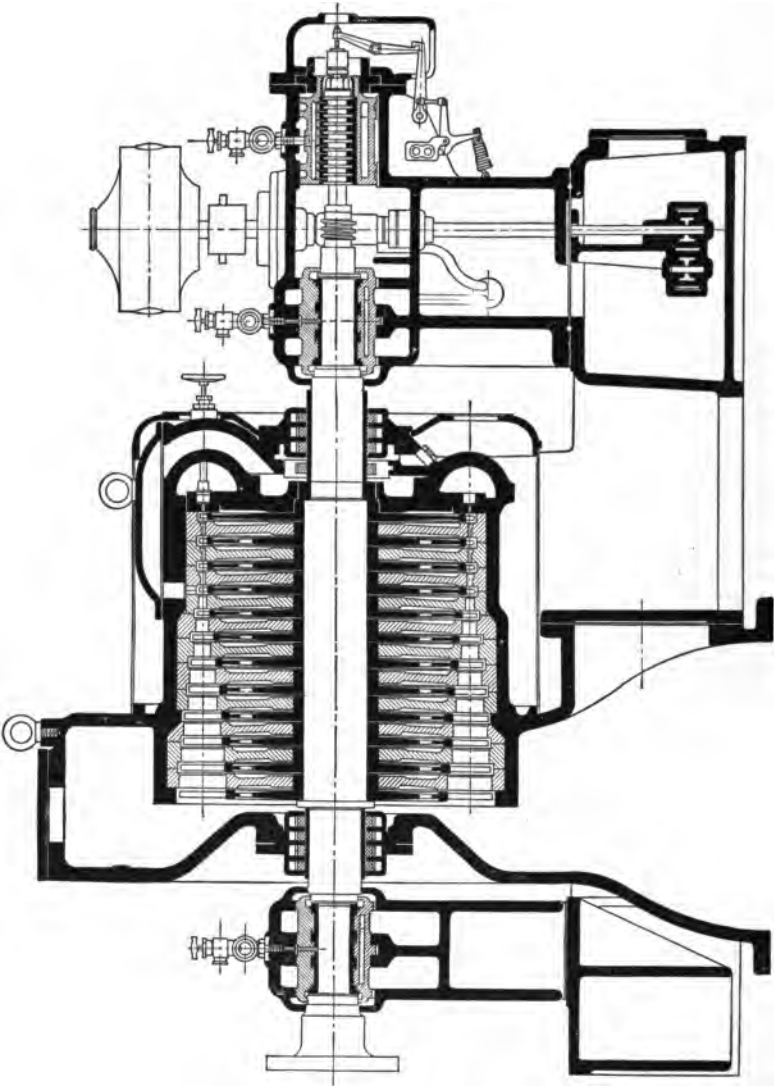
FIG. 169. De Laval Pressure-stage Turbine.
