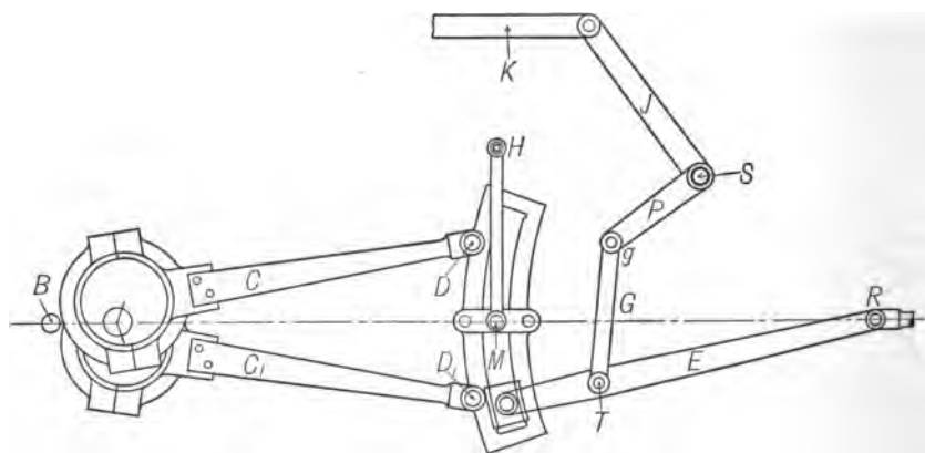
FIG. 148. Gooch Link.
