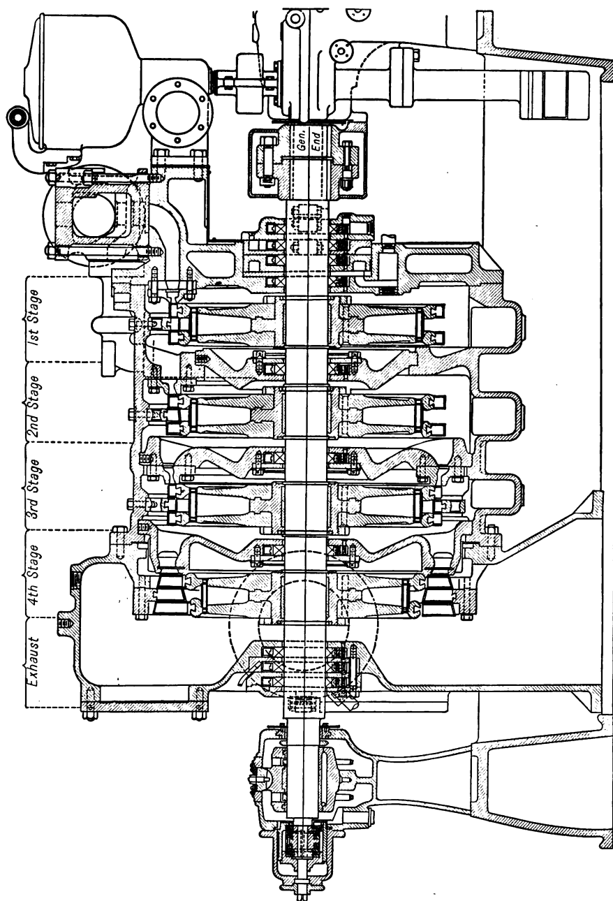
FIG. 172. Curtis Turbine.
