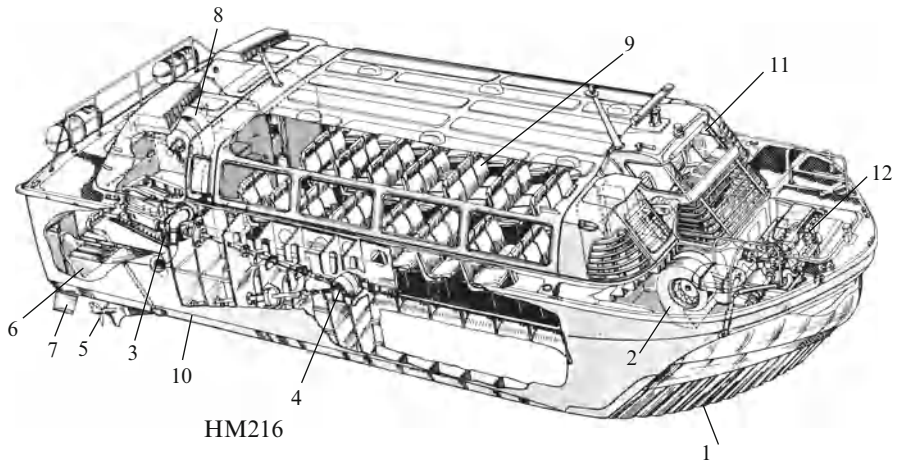
Fig. 2.45 Hovermarine HM2 Cutaway
