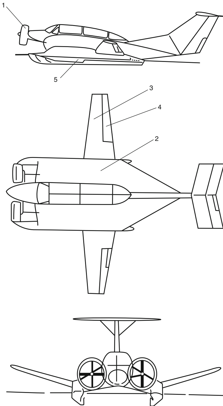
Fig. 3.19 Ivolga 3 view
