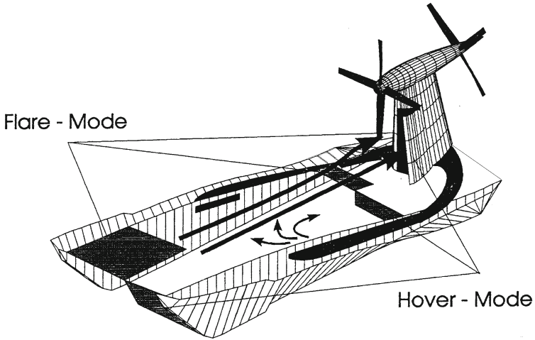
Fig. 3.10 Hoverwing diagram
