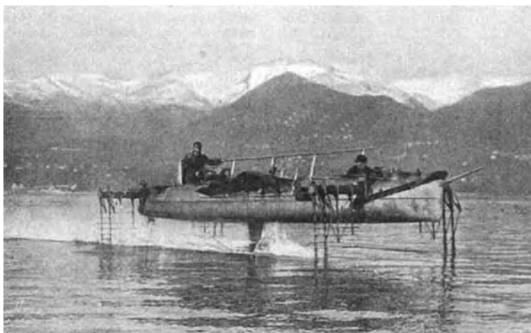
Fig. 5.2 Forlanini hydrofoil from 1906 on lake Maggiore
