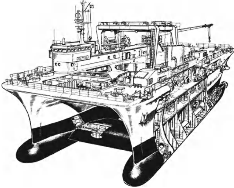
Fig. 6.33 Duplus SWATH
