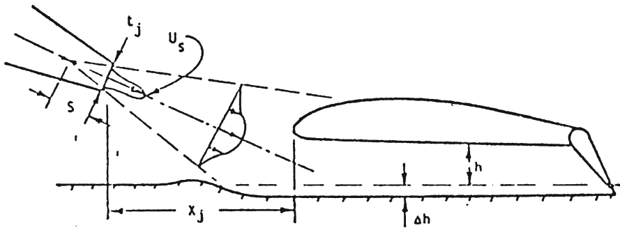
Fig. 3.17 DACC/PAR diagram
