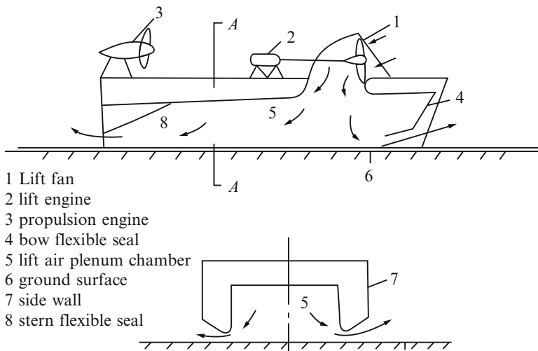
Fig. 2.44 Sidewall SES plenum chamber principle
