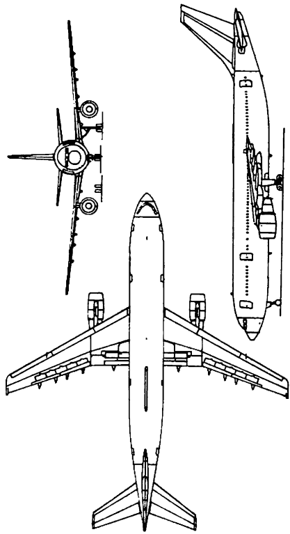
b) AIRBUS A 300 B4
