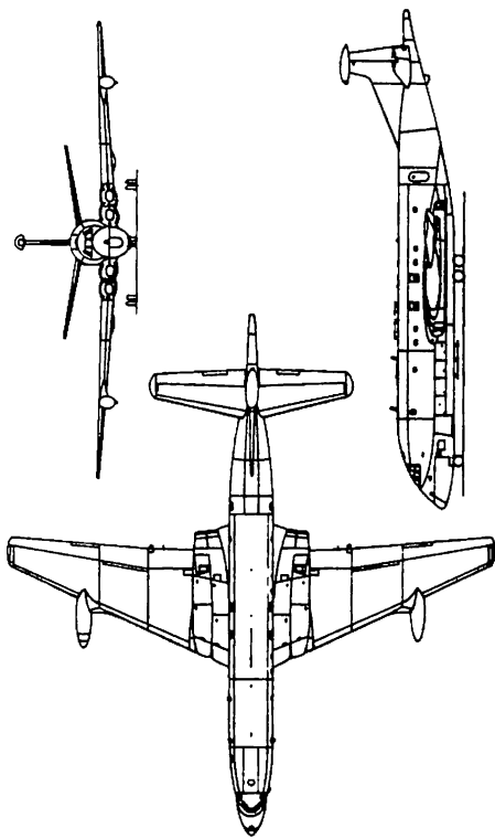
b) BAE HS NIMROD MR. MK 1
