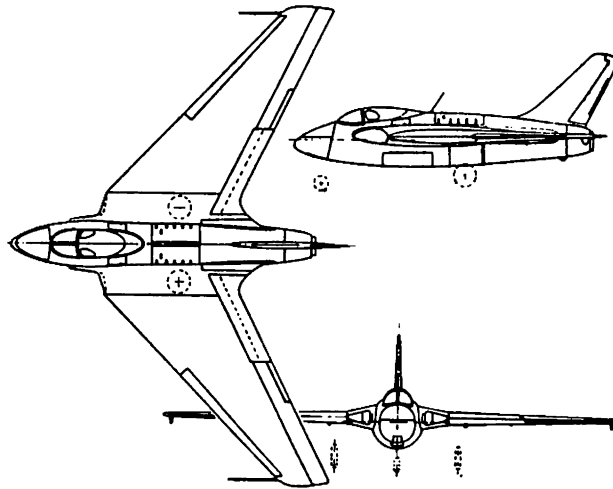
Figure 3.53 DeHavilland DH 108
