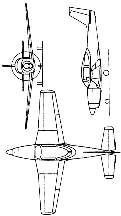
b) INTERCEPTOR 400
