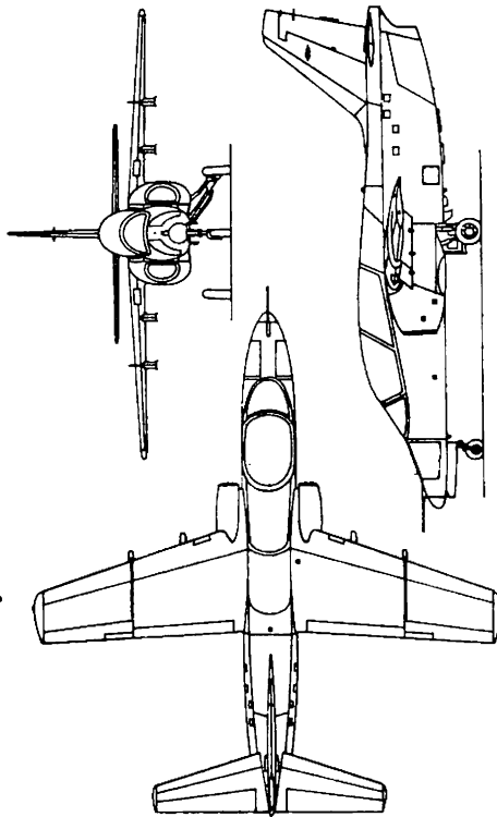
c) SIAI - MARCHETTI S.211
